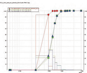
Exemple courbe granulométrique sur 3 filtres
